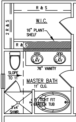
OPTIONAL MASTER BATH
