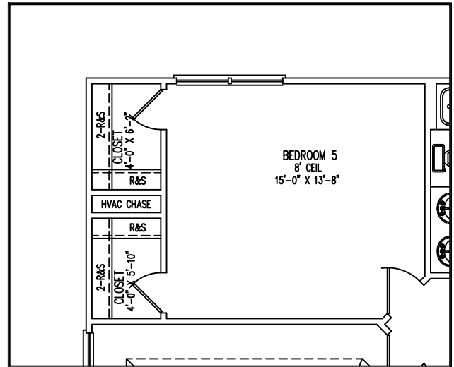
OPTIONAL BEDROOM 5
